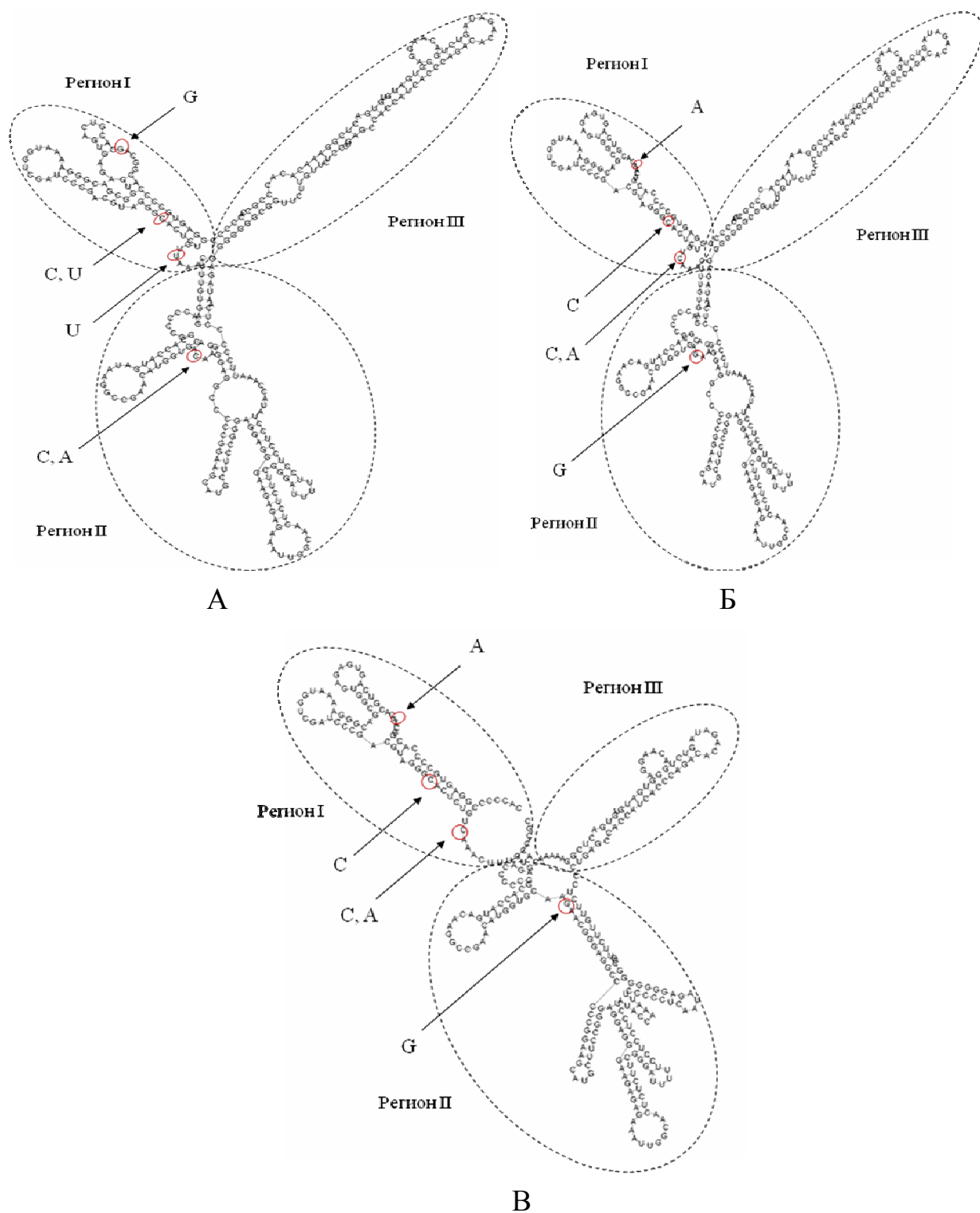
Рис. 2. Модели вторичной структуры корового элемента 3'НТР исследуемых штаммов. А – структура, сформированная последовательностями штаммов Primorye-86, Primorye-90, Primorye-212, Primorye-270, Primorye-253 и Primorye-332 и Primorye-18; Б – структура, сформированная последовательностями штаммов Kavalerovo, Glubinnoe и Sofjin-NO; В – структура, сформированная последовательностями штаммов Primorye-89, Dalnegorsk и Svetlogorie. Стрелками показаны группоспецифичные нуклеотидные замены. Пунктирными линиями выделены участки структуры, формирующие Регионы I, II и III корового элемента 3'НТР.
